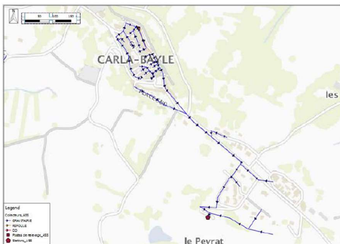
FIGURE 10 : PLAN DES RESEAUX D'ASSAINISSEMENT DES EAUX USEES DE LA COMMUNE DE CARLA BAYLE BOURG
