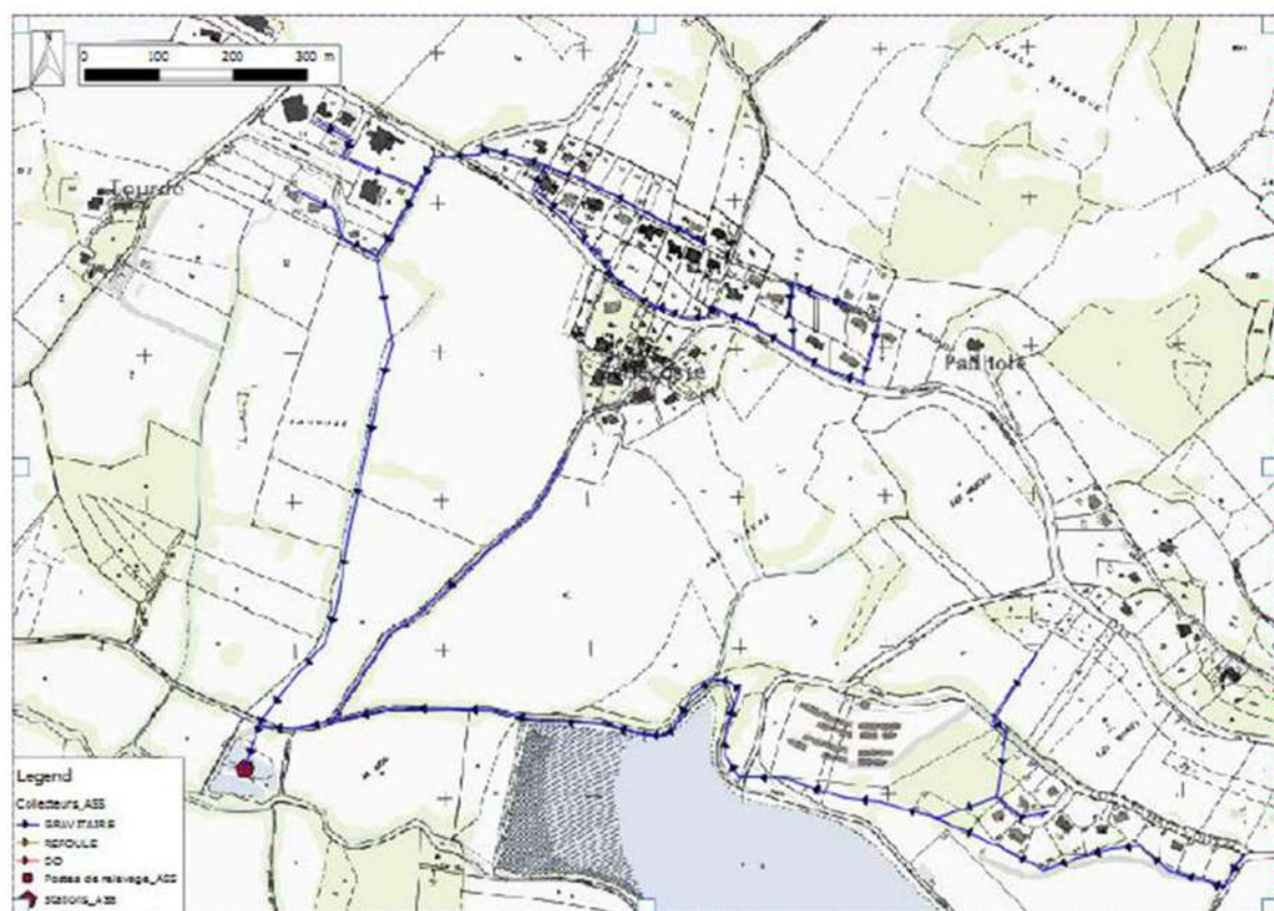
FIGURE 13 : PLAN DES RESEAUX DES EAUX USEES SUR LA COMMUNE DE CARLA BAYLE LAC
